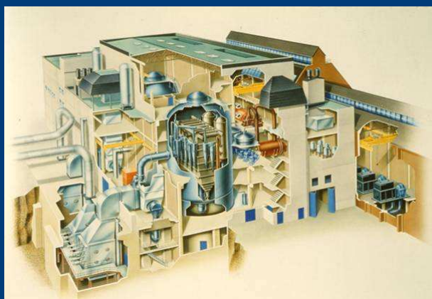
PFBC - trycksatt fluidiserad bädd 2 x 230 t/h (ca 420 MWth)
